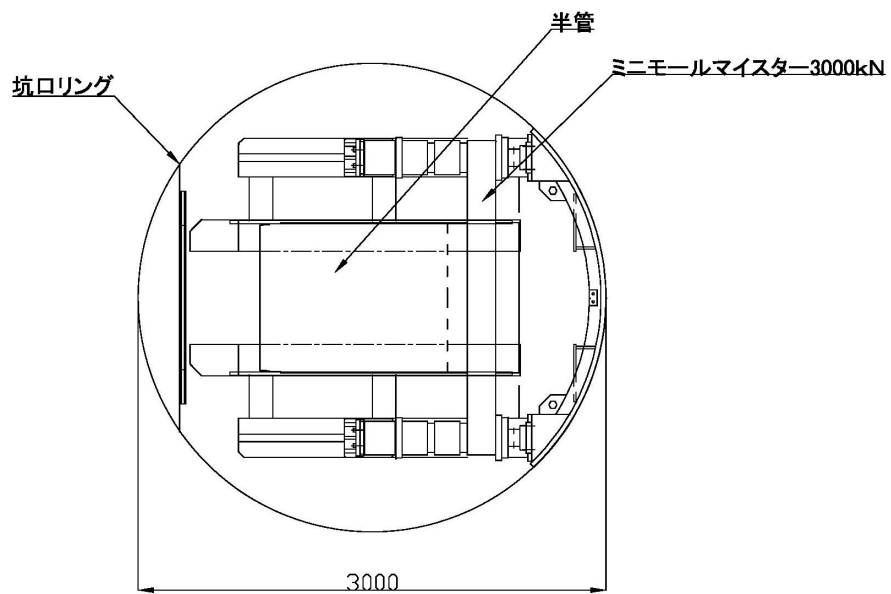
図 2-1 呼び径 800~1000
