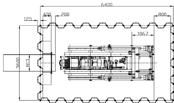
鋼管 800 T型モールマイスター（引戻し時） 鋼管切断対応
