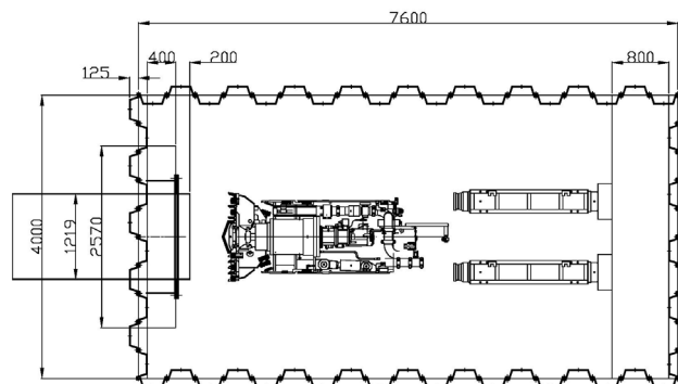
鋼管 1200 多段ジャッキ（引戻し時） 鋼管切断対応
