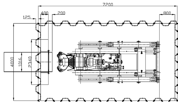
鋼管 1000 T型モールマイスター（引戻し時） 鋼管切断対応
