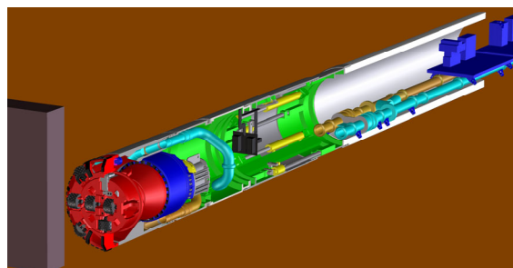
図 13-2 制御機器・送排泥管撤去
