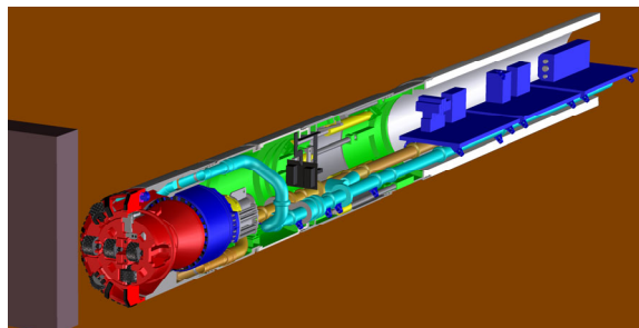
図 13-1 掘進機到達
