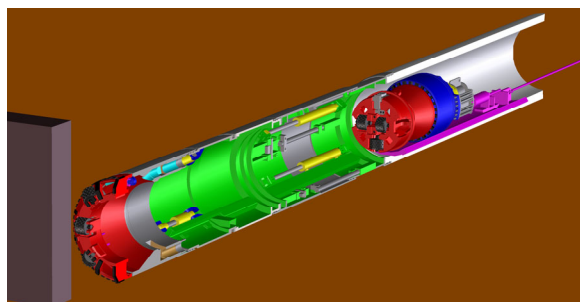
図 13-3 掘進機引戻し
